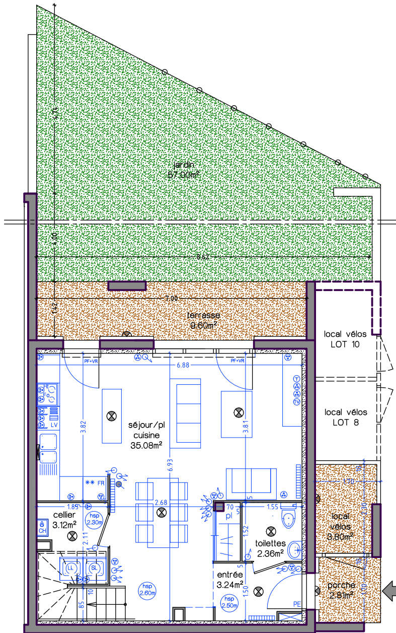
REZ DE CHAUSSEE
